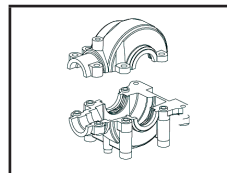
No. 505075 Getriebegehäuse Gear box
