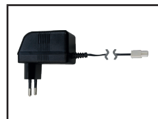
No. 505270 Tam 230 V 12 V 350 mAh Ladegerät Charger
