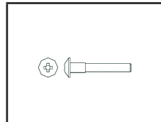
No. 505054 3 x 35 | 3 x 26 | 3 x 22 mm Querlenkerstifte oben/außen Suspension arm shaft set
