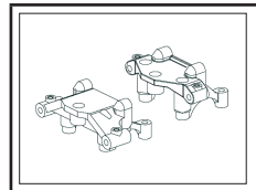
No. 505078 Stoßdämpferhalter Shock mount
