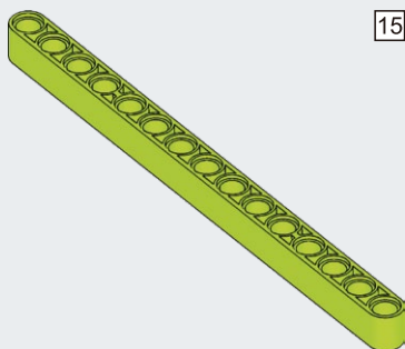
3x JJ60100008
